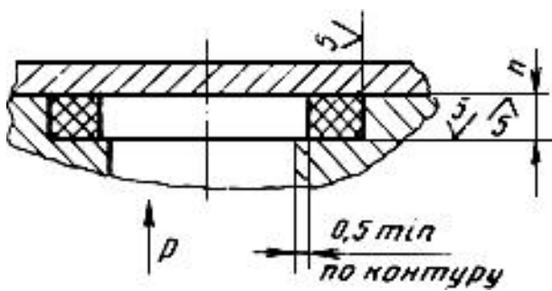
Черт.8
